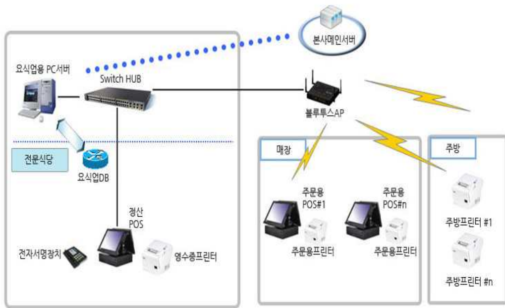
[그림 3-4] 레스토랑 POS 시스템 구성도 출처: http://www.brain21c.co.kr
